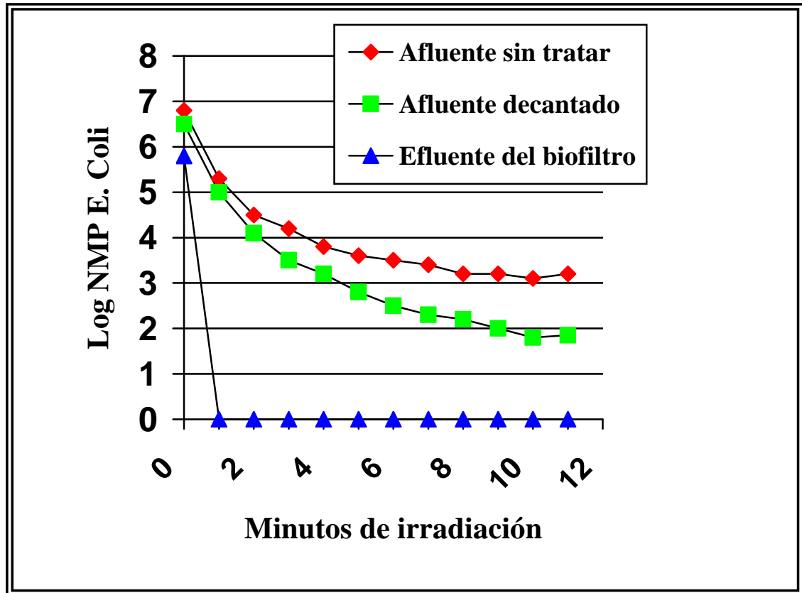
Figura 2. Tiempo de decaimiento bacteriano por radiación ultra violeta
