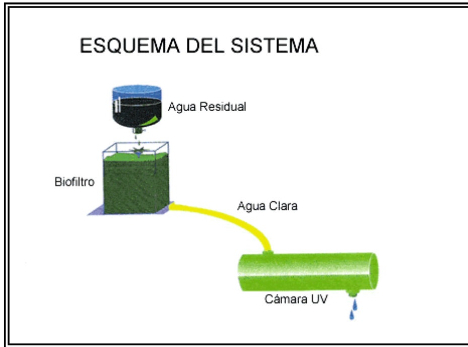
Figura 1. Esquema del Sistema Tohá
