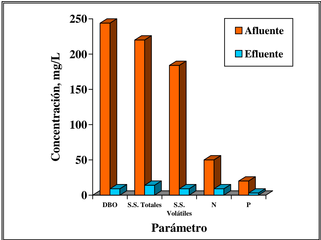
Figura 3. Eficiencia del biofiltro: valores máximos y mínimos de los parámetros de DBO, sólidos suspendidos totales, sólidos suspendidos volátiles, nitrógeno total y fósforo total.
